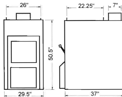
DIMENSIONS
