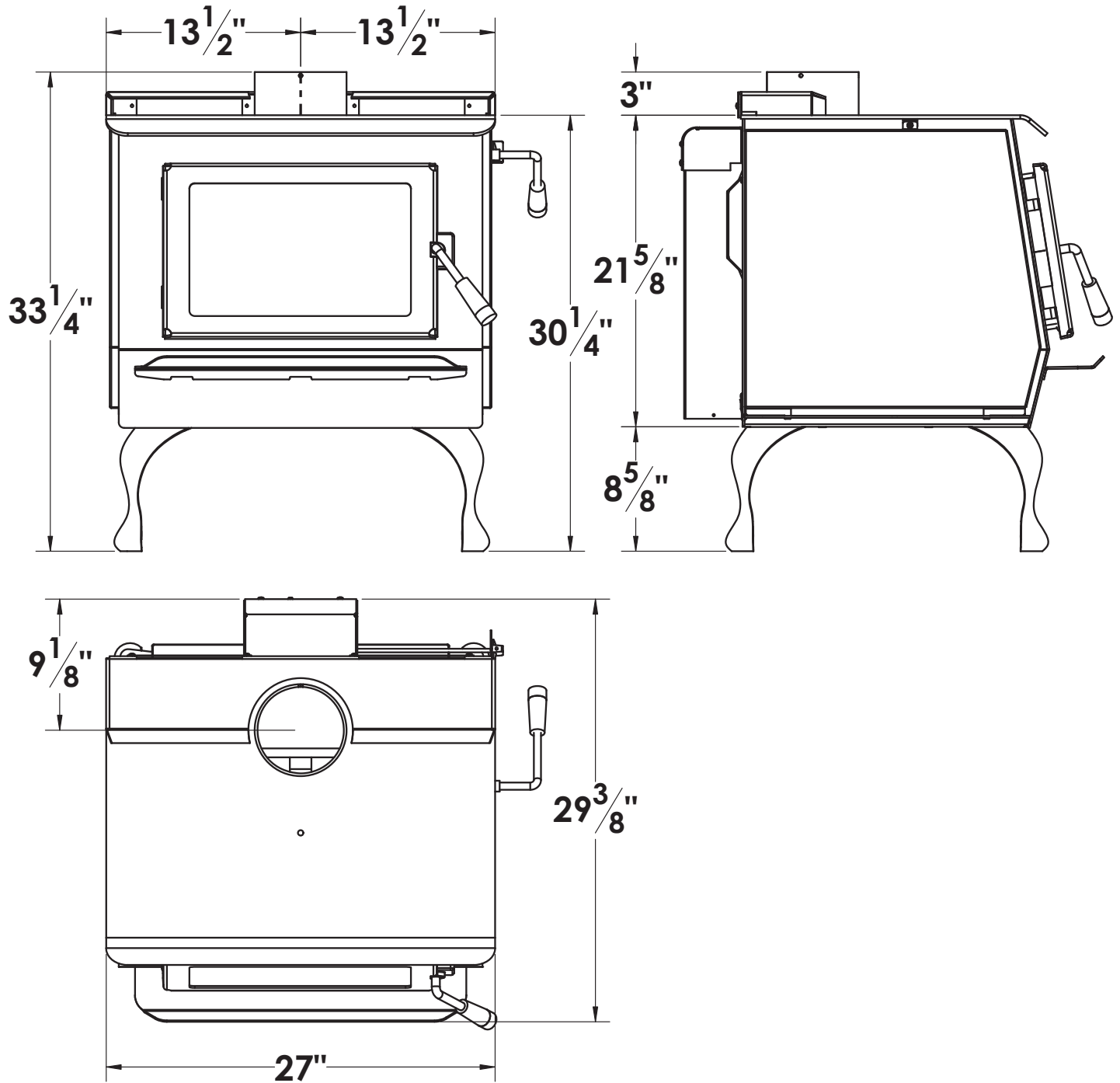
PE32 AVEC ENSEMBLE DE PATTES PARLOR (S.Z1713)
