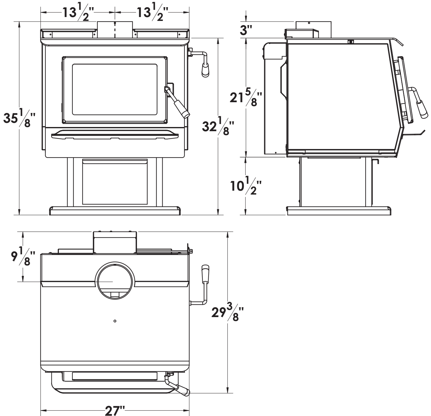
PE32 AVEC PIÉDESTAL ULTRA (S.Z3903)
