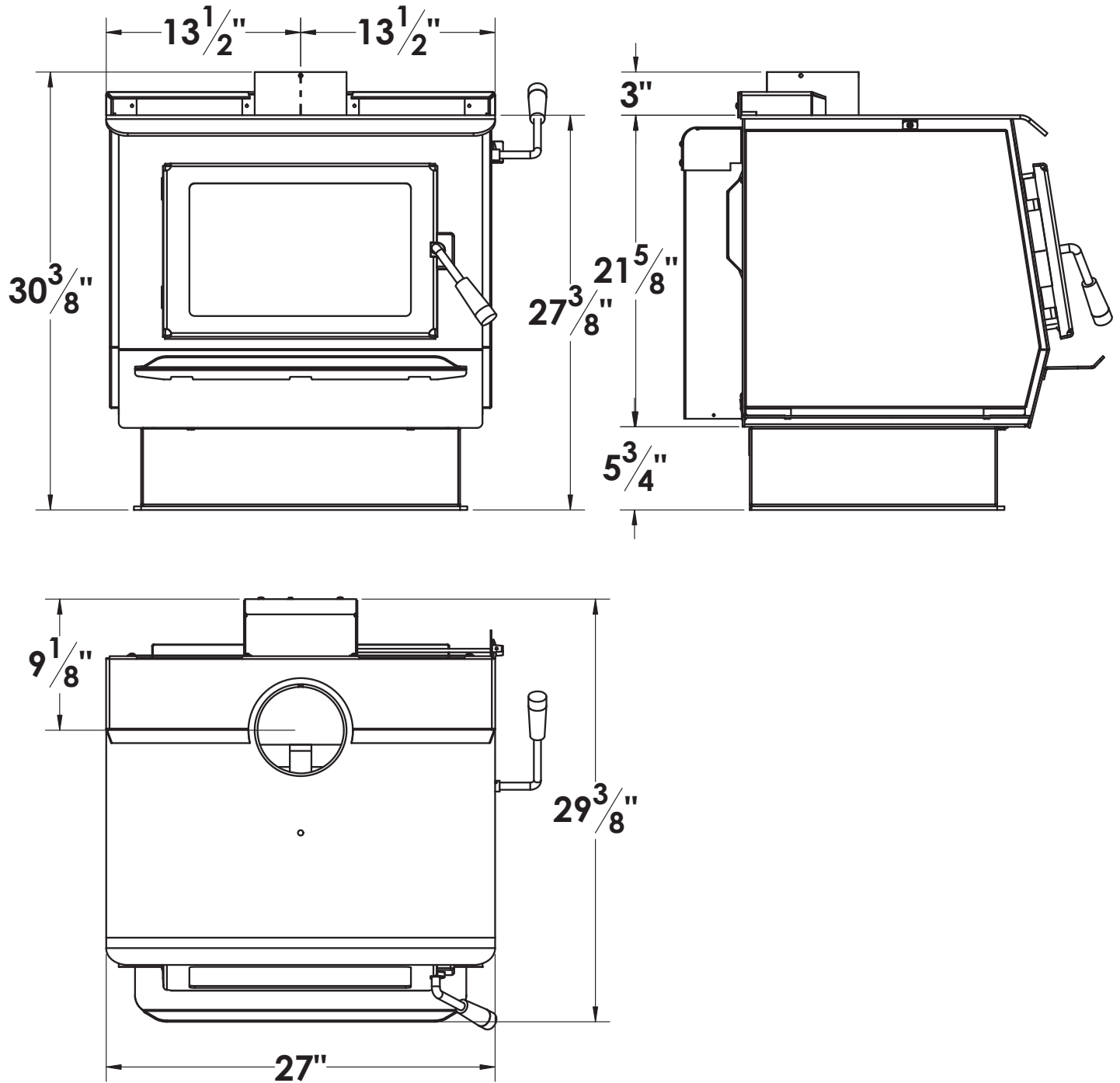
PE32 AVEC BASE CLASSIQUE (S.Z4815)
